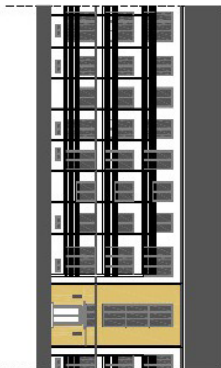
WESTANSICHT OSTFLÜGEL
